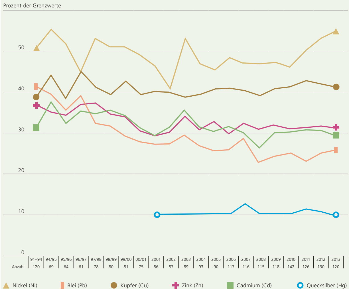
Abb. 7: Schwermetallgehalte der Zürcher Komposte und Gärgut 1991 bis 2013 in Prozenten der Grenzwerte (Median- oder Zentralwerte)
